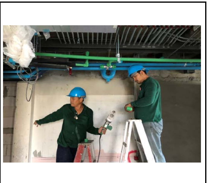
Activity เดินท่อน้ำดี,นำทิ่งห้องตัวอย่าง No.20,24 Floor 8 Date : 27 July 2563
