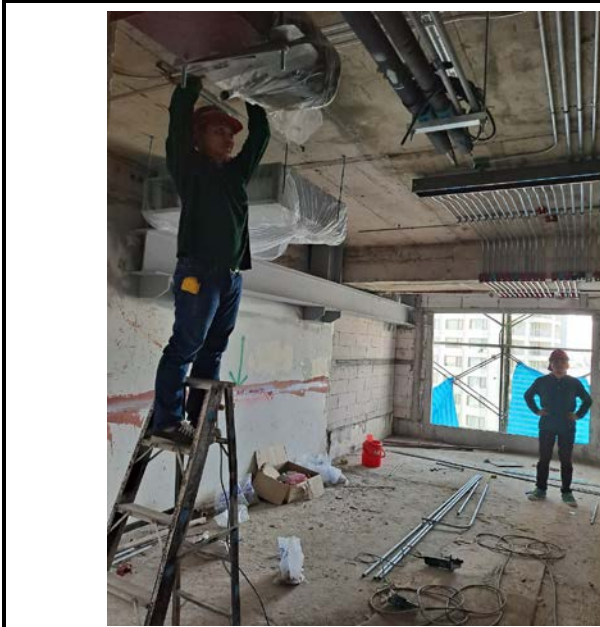
Activity เดินท่อไฟฟ้าเหนือฝ้าบริเวณห้องพัก Floor 11 Date : 6 October 2563
