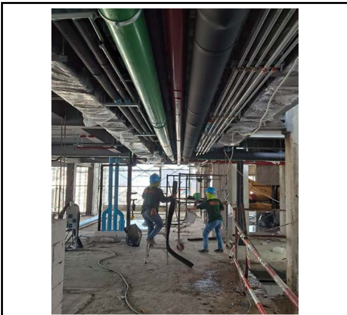
Activity หุ้มฉนวนท่อ CW,HW บริเวณ Corridor Floor 16 Date : 6 October 2563
