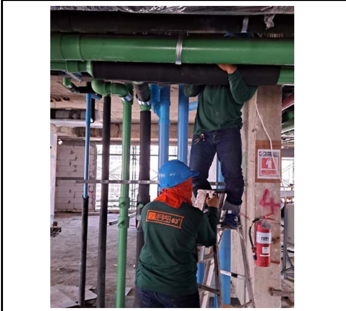
Activity หุ้มฉนวนท่อ CW,HW บริเวณ Corridor Floor 12 Date : 6 October 2563
