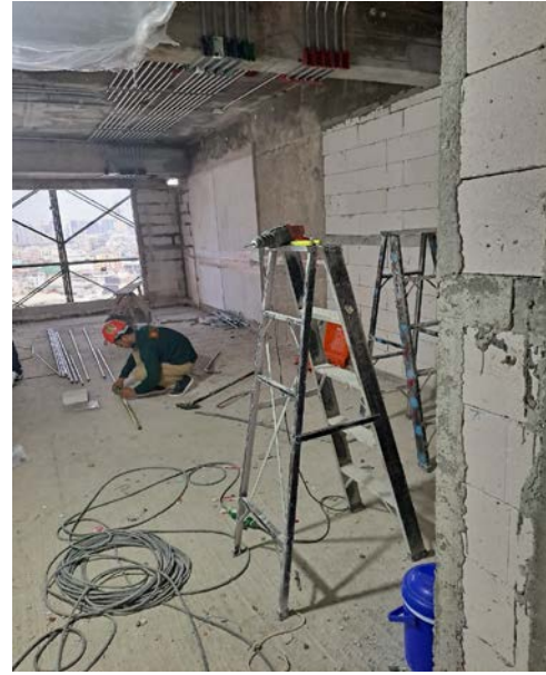
Activity เดินท่อไฟฟ้าเหนือฝ้าบริเวณห้องพัก Floor 14 Date : 23 October 2563
