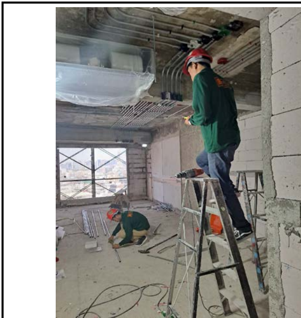
Activity เดินท่อไฟฟ้าเหนือฝ้าบริเวณห้องพัก Floor 14 Date : 23 October 2563
