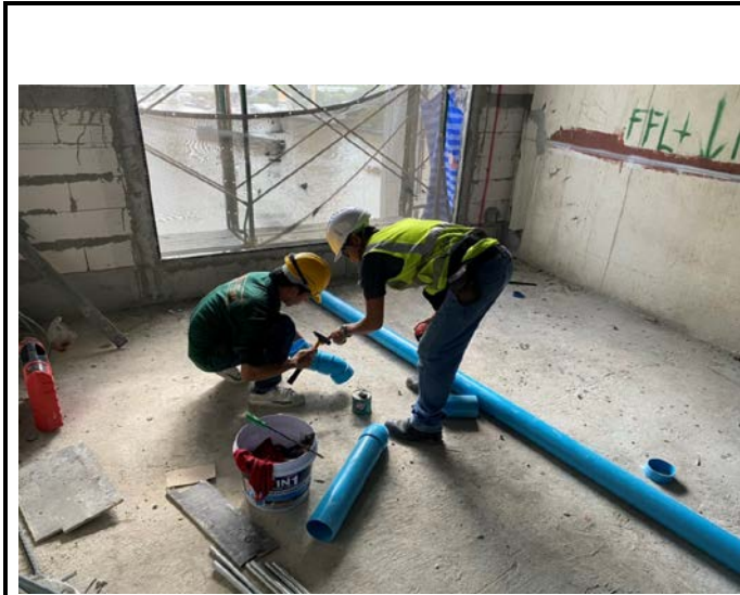
Activity เดินท่อดูดอากาศบริเวณห้องพัก Floor 11 Date : 2 November 2563
