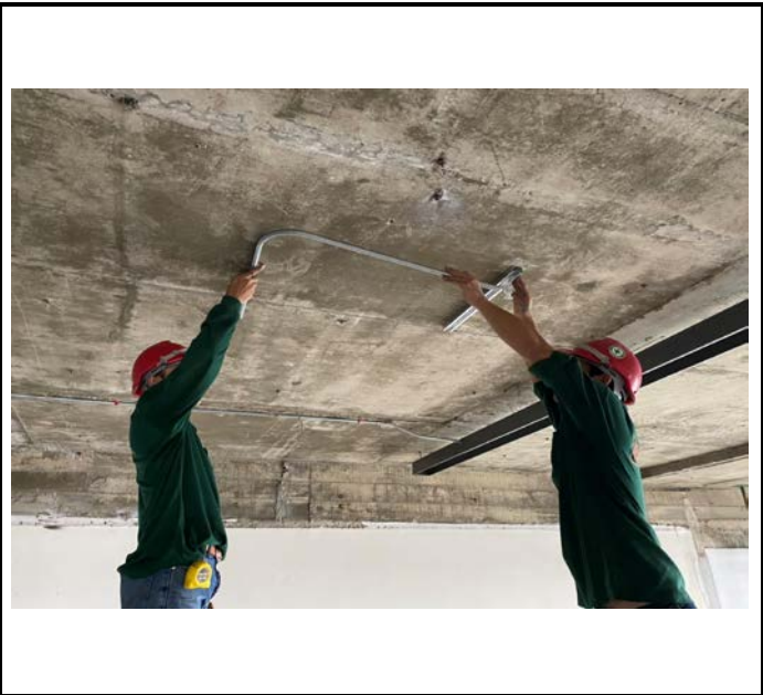
Activity เดินท่อไฟฟ้าเหนือฝ้าบริเวณห้องพัก Floor 14 Date : 2 November 2563
